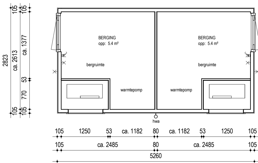
PLATTEGROND
