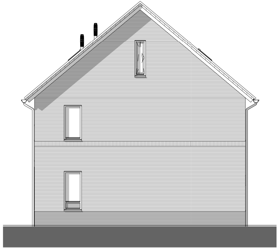
Rechter gevel 1 : 100
