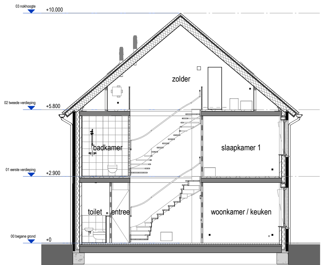
Doorsnede 1 : 100
