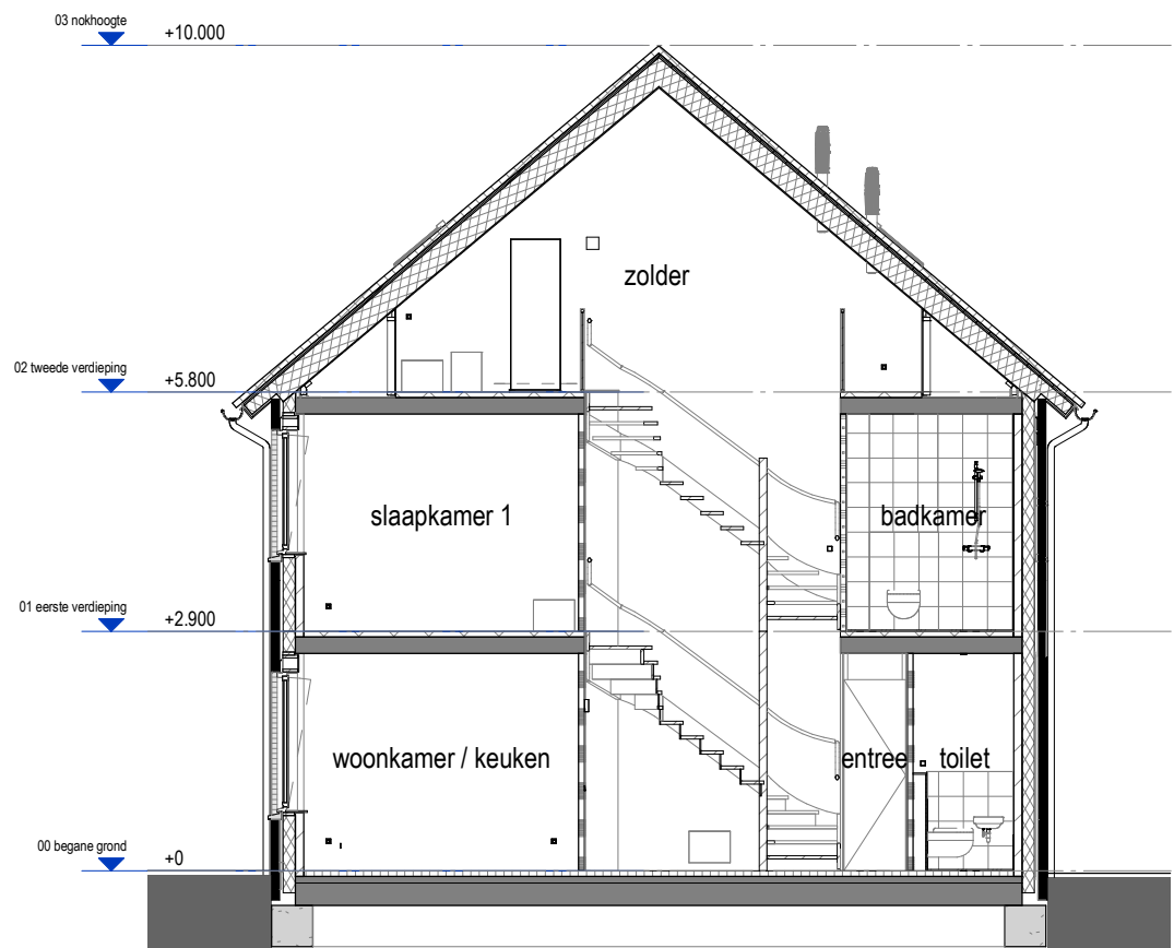
Doorsnede 1 : 100
