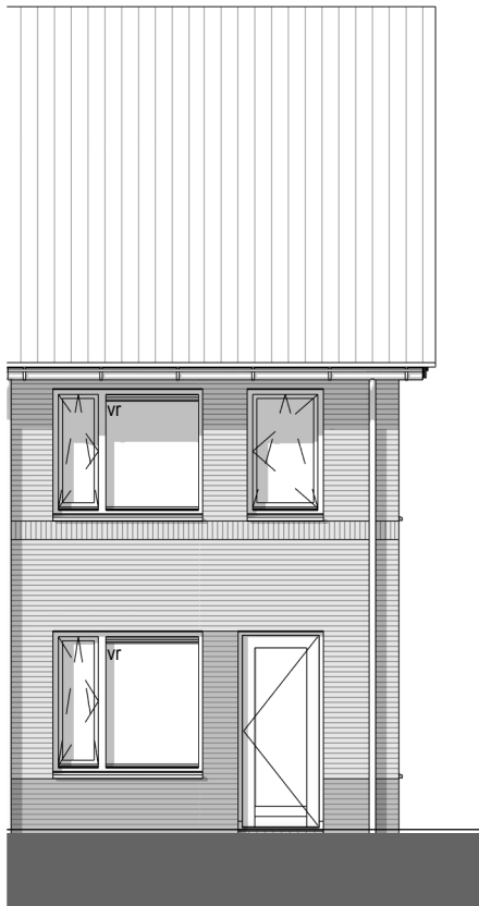
Achtergevel 1 : 100
