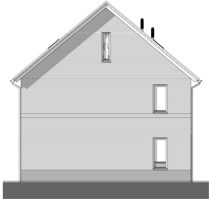
Zijgevel 1 : 100
